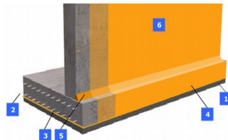
Rys. 1. Kompleksowa izolacja podziemnej części z użyciem Hydrostopu: 1-chudy beton; 2-zbrojenie; 3-płyta fundamentowa; 3-warstwa Hydrostopu-Mieszanki równomiernie rozsypana; 4-bok płyty uszczelniony Hydrostopem-Mieszanką Profesjonalną; 5-klin z Hydrostopu-Zaprawy Wodoszczelnej; 6-bok ściany uszczelniony Hydrostopem-Mieszanką Profesjonalną.
